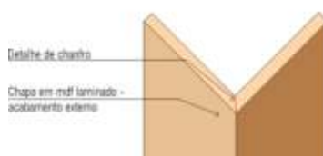
fig.: detalhe acabamento de encontro com angulação de placas de MDF laminado
